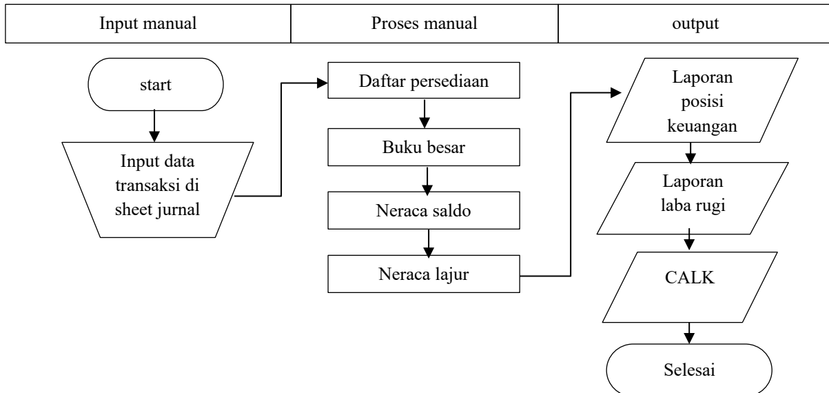
Gambar 1. Siklus Pencatatan Akuntansi Microsoft Excel
